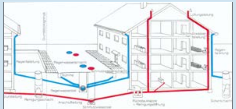
Illustration Trennsystem
